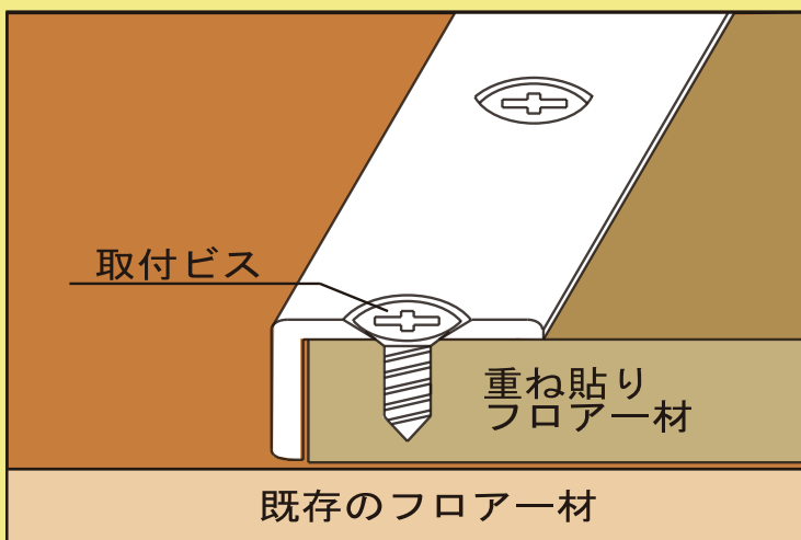
[施工断面図]
