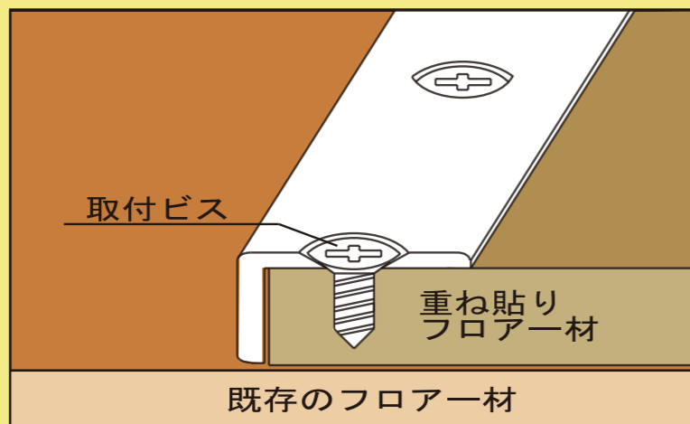
〔施工断面図〕
