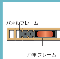
取り付け断面図
