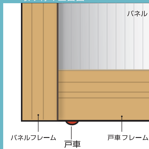
取り付け正面図
