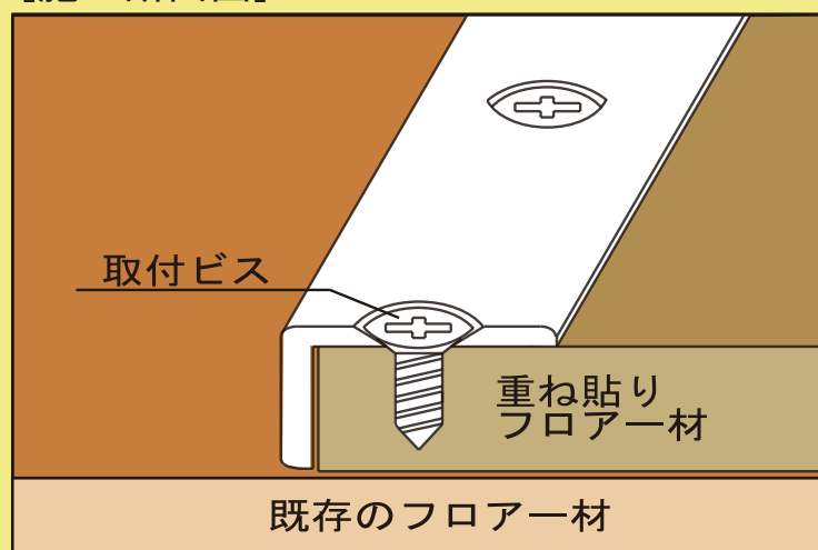
〔施工断面図〕
