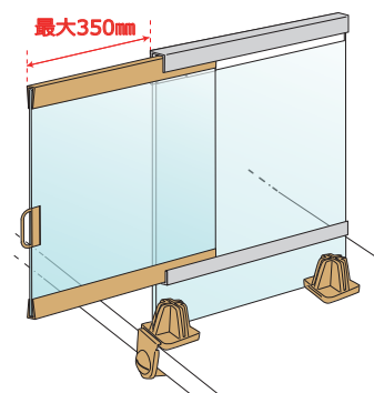
パネル最大引き出し時(高さ) 600mm×(横幅) 800mm
