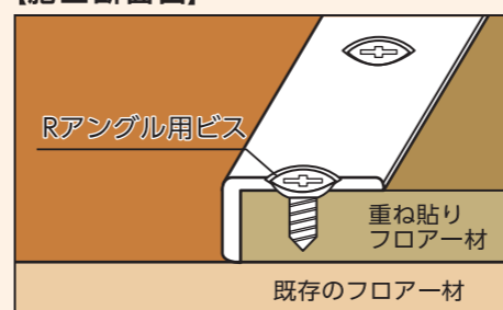
【施工断面図】
