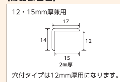
【商品断面図】
