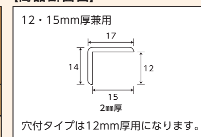
【商品断面図】
