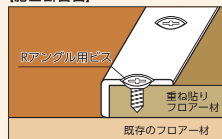
【施工断面図】
